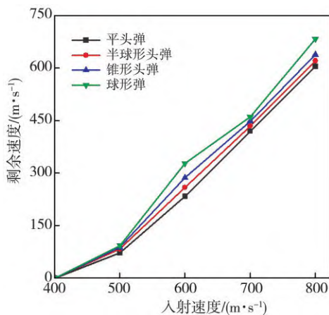
图 8 不同入射速度下弹体剩余速度
