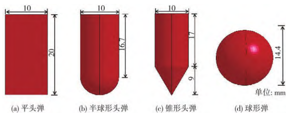
图 7 不同弹头形状子弹尺寸
