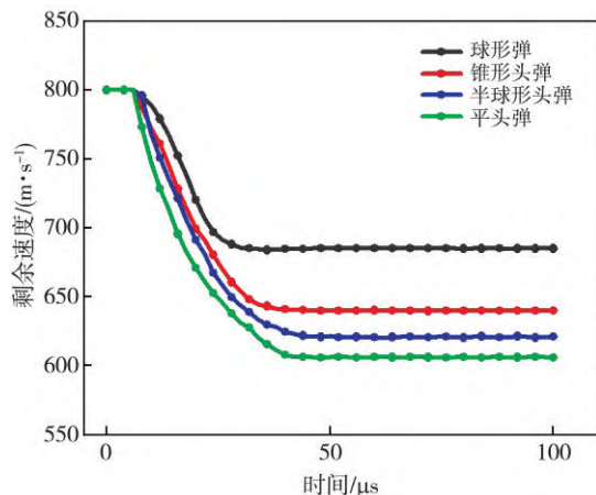
图 9 不同弹头形状弹体的速度变化
