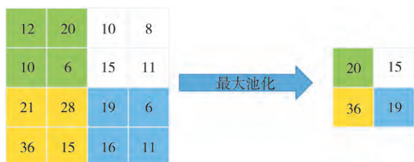
图2 最大池化
