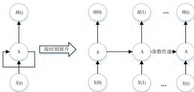
图3 RNN结构展开图
