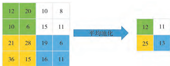
图1 平均池化
