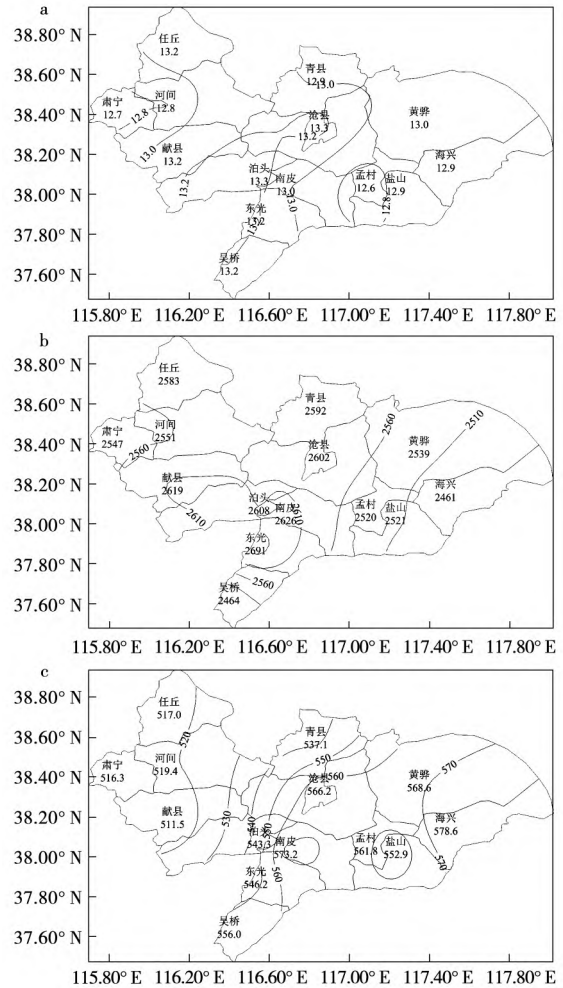
图 1 1973—2022 年沧州市平均气温(a)、日照时数(b)和降水量(c)的空间分布
