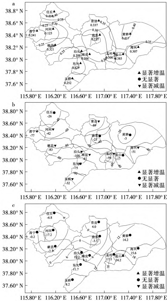
图 2 1973—2022 年沧州市平均气温(a)、日照时数(b)、降水量(c)的气候倾向率和 MK 趋势检验空间分布注:气温倾向率单位为 ^{\circ}\text{C}\cdot(10\text{ a})^{-1} ;日照时数倾向率单位为 \text{h}\cdot(10\text{ a})^{-1} ;降水量倾向率单位为 \text{mm}\cdot(10\text{ a})^{-1} 。
