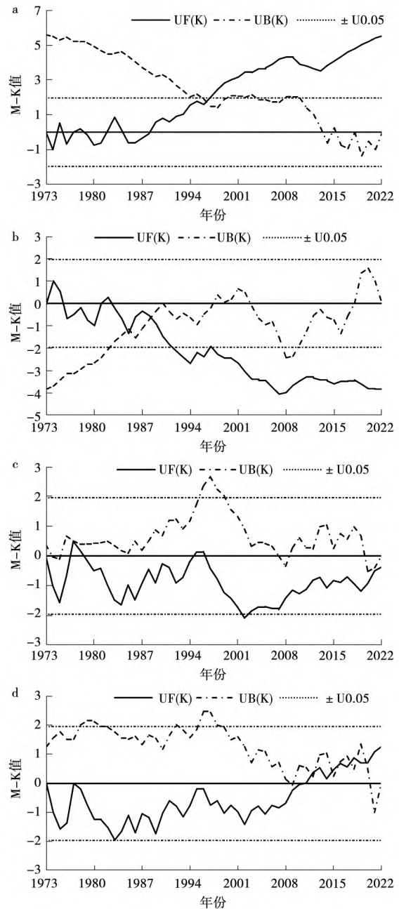
图 3 1973—2022 年沧州市平均气温(a)、日照时数(b)、中西部县市降水量(c)和其他县市降水量(d)的 MK 突变检验注:中西部县市包括沧县、任丘、肃宁、河间和献县;其他县市包括除沧县、任丘、肃宁、河间和献县外的县市。下同。
