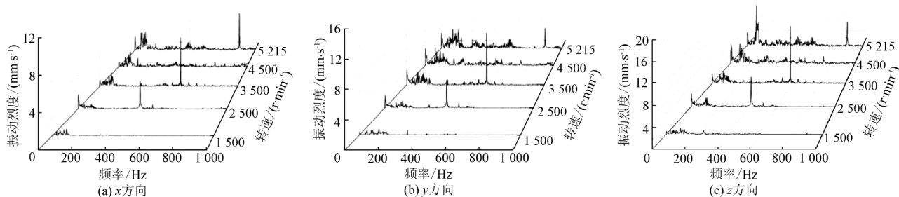
图9 不同转速时驱动端轴承体 x 、 y 、 z 方向的频谱图
