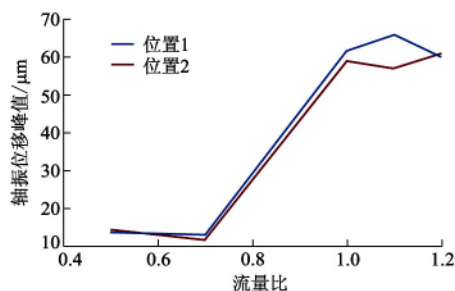
图5 不同流量比下的轴振测试结果
