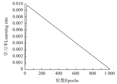
图 6 学习率曲线
