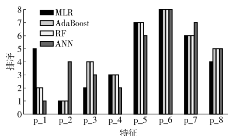
图 6 基于土壤因素的建模特征重要性排序
