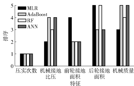
图 5 基于机械因素的建模特征重要性排序
