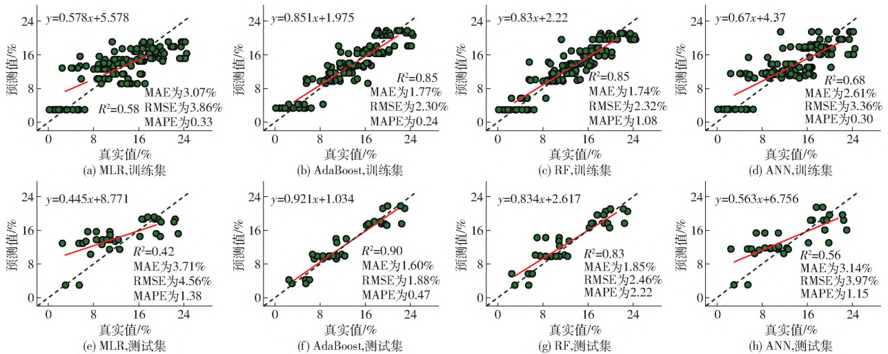
图 2 基于机械因素的大豆产量影响预测模型效果拟合曲线
