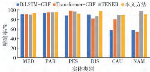
图 3 各实体精确率对比
