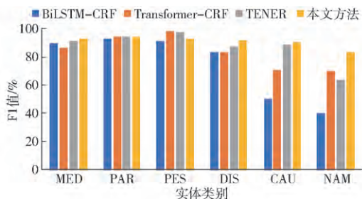
图 5 各实体 F1 值对比
