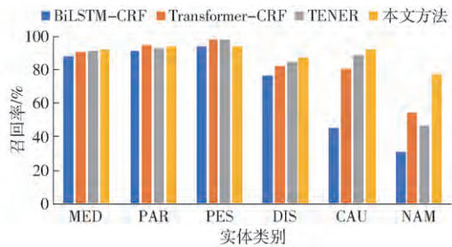
图 4 各实体召回率对比
