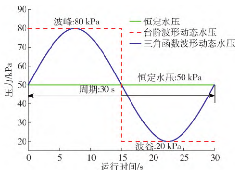
图2 水压示意图
