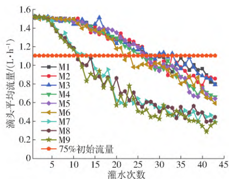
图3 不同水压模式下滴头平均流量与灌水次数的关系
