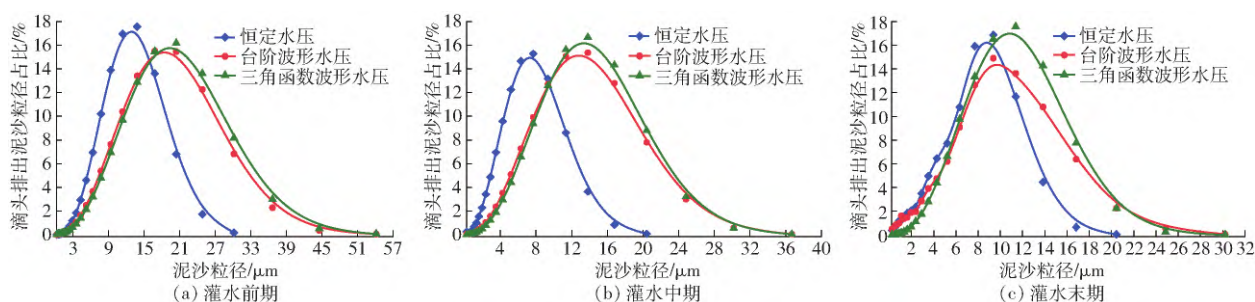
图9 不同水压模式下滴头排出泥沙粒径变化曲线
