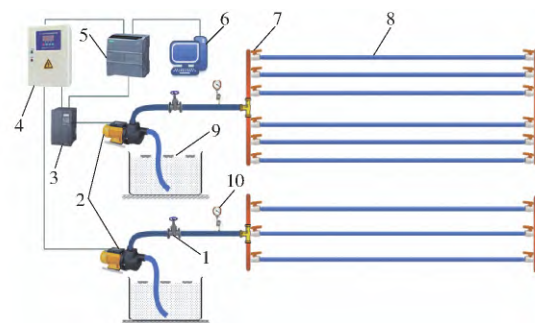
图1 滴灌系统试验平台
