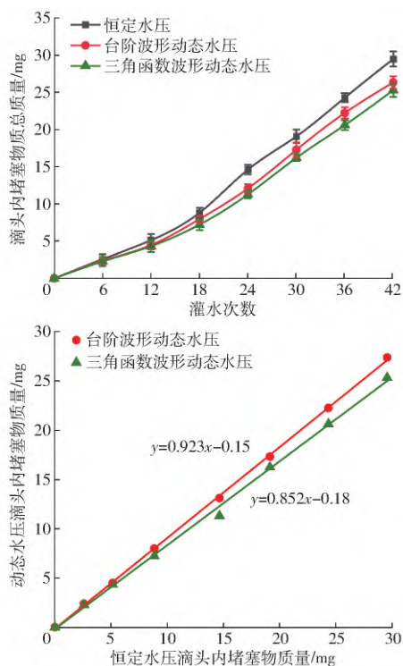
图7 滴头内堵塞物质的总质量和线性回归曲线
