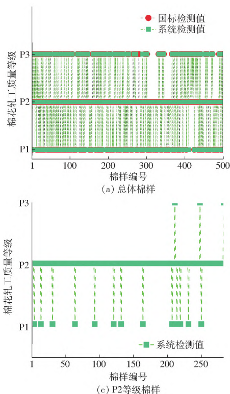
图 10 系统检测与国标检验结果对比
