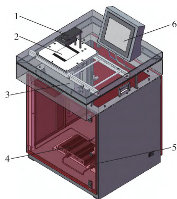
图 1 棉花轧工质量视觉检测系统结构图
