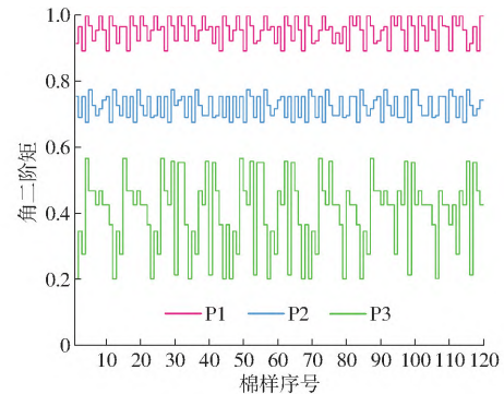
图 7 轧工质量实物标准的纹理特征
