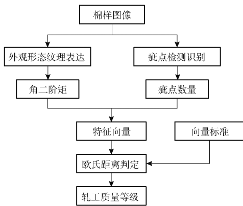
图4 检测算法流程图
