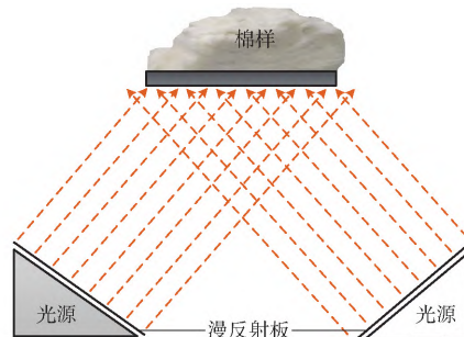
图 2 光照系统原理图
