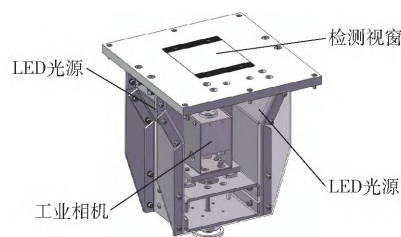
图 3 图像采集机构
