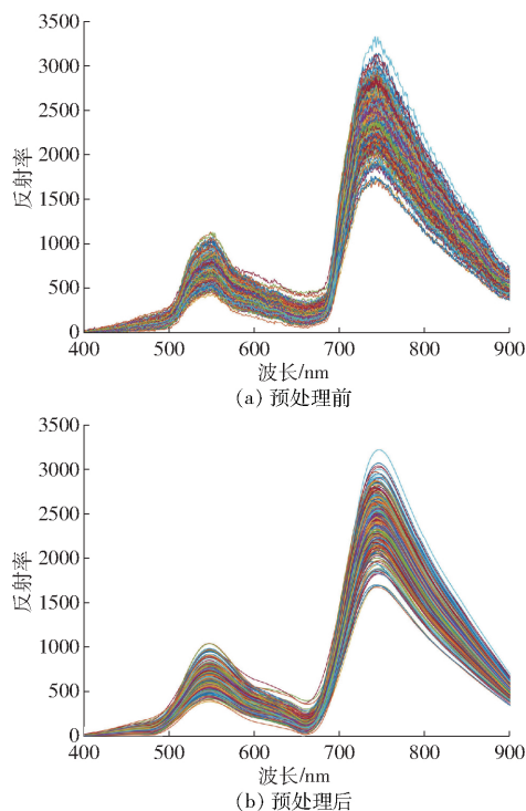
图6 S-G 平滑预处理前后光谱图像对比
