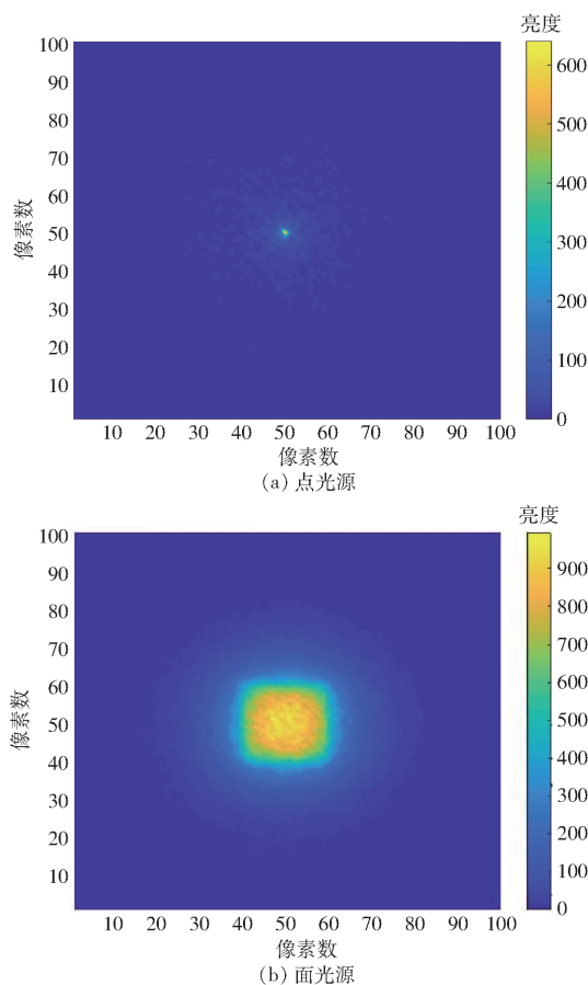
图3 仿真光子分布图
