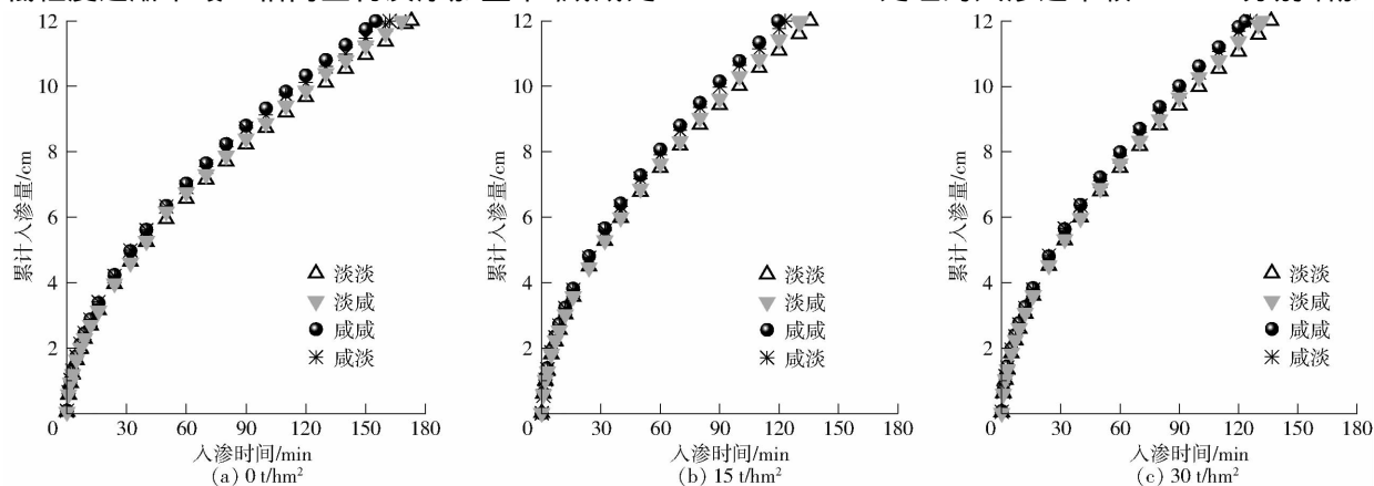
图3 咸淡轮灌和生物炭添加下累计入渗量随时间的变化曲线
