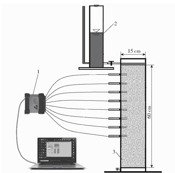
图1 试验装置示意图
