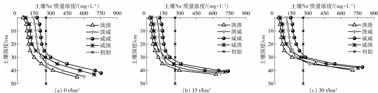
图8 咸淡轮灌和生物炭添加下土壤剖面 \text{Na}^+ 含量分布
