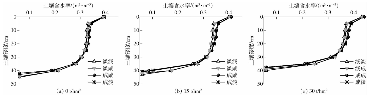
图5 咸淡轮灌和生物炭添加下土壤剖面含水率分布
