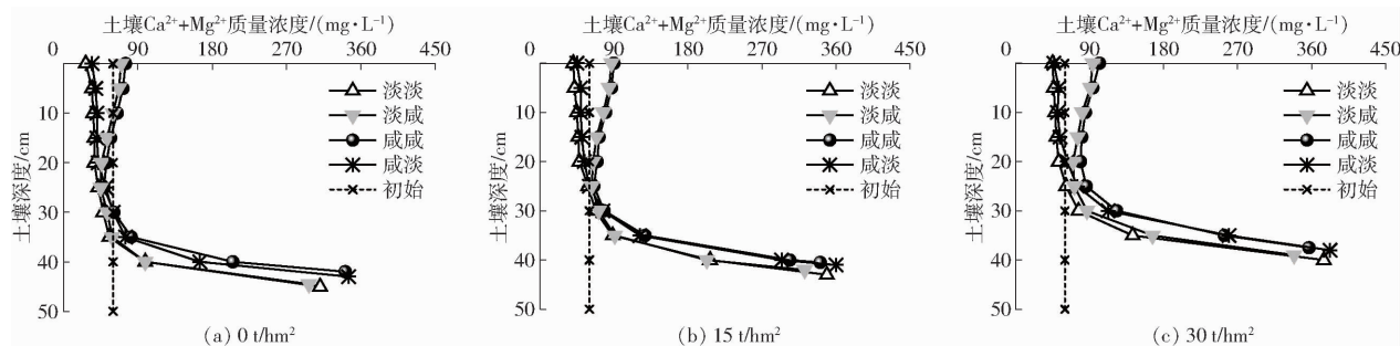
图9 咸淡轮灌和生物炭添加下土壤剖面 \text{Ca}^{2+} 和 \text{Mg}^{2+} 含量分布
