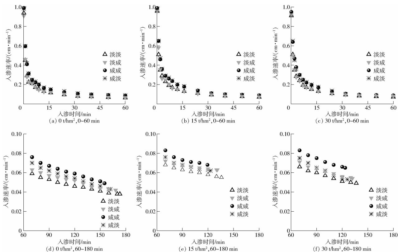
图4 咸淡轮灌和生物炭添加下入渗速率随时间的变化曲线
