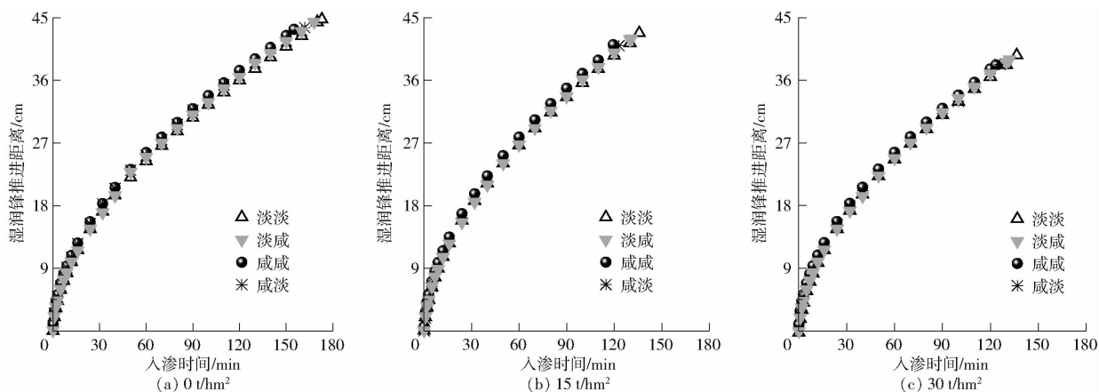
图2 咸淡轮灌和生物炭添加下湿润锋推进距离随时间的变化曲线
