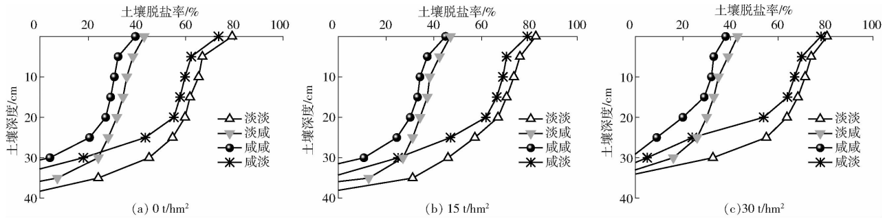
图7 咸淡轮灌和生物炭添加下土壤剖面脱盐率分布
