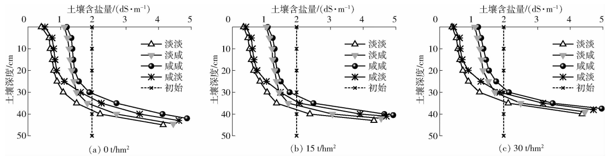
图6 咸淡轮灌和生物炭添加下土壤剖面含盐量分布
