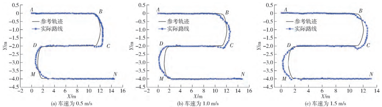
图 8 实车试验路径跟踪曲线
