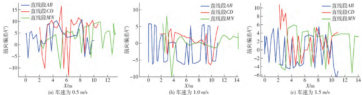
图 10 实车试验直线航向偏差
