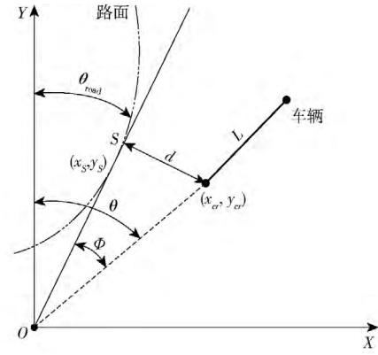
图 2 路径跟踪误差模型
