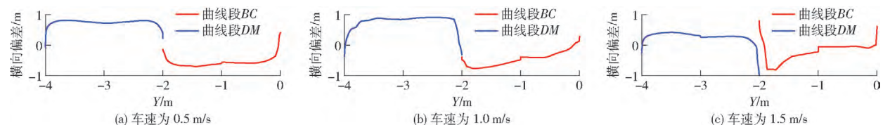
图 11 实车试验曲线横向偏差
