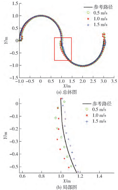
图 5 曲线参考轨迹与实际轨迹
