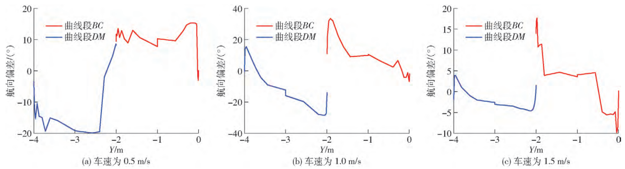
图 12 实车试验曲线航向偏差 Fig. 12 Heading deviation of real vehicle test curves
