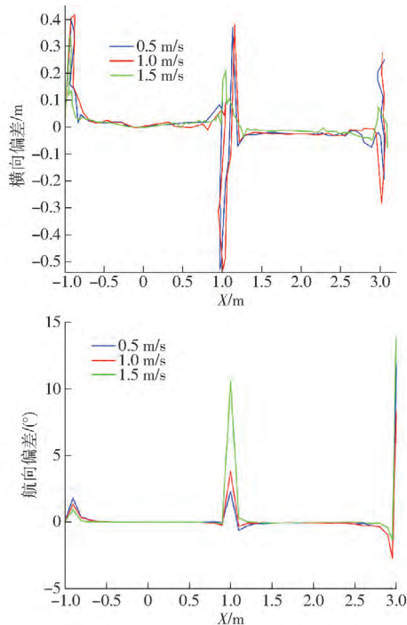
图 6 3 种速度下横向、航向偏差曲线(曲线跟踪)
