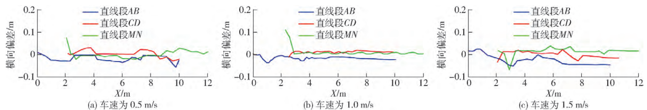
图 9 实车试验直线横向偏差
