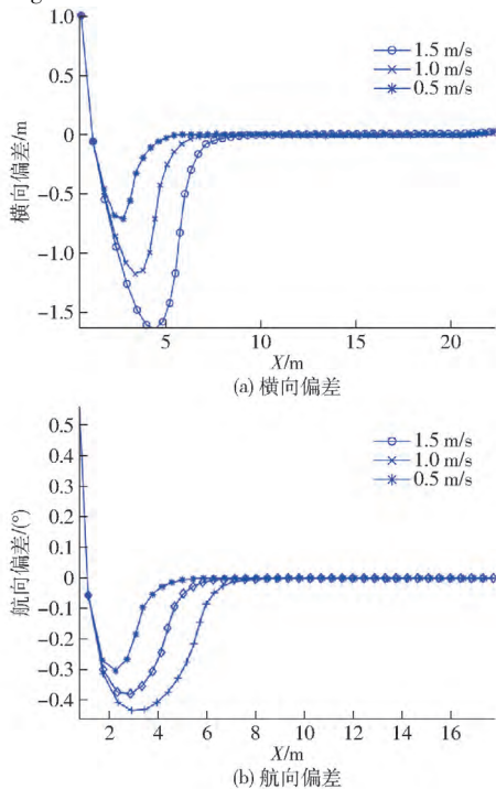
图 4 3 种速度下横向、航向偏差曲线(直线跟踪)
