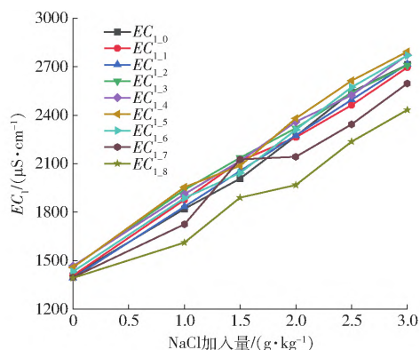
图2 EC_1 与 NaCl 加入量关系
