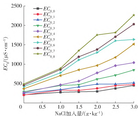
图1 EC_0 与 NaCl 加入量关系
