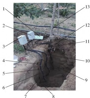
图7 大田试验传感器布置示意图
