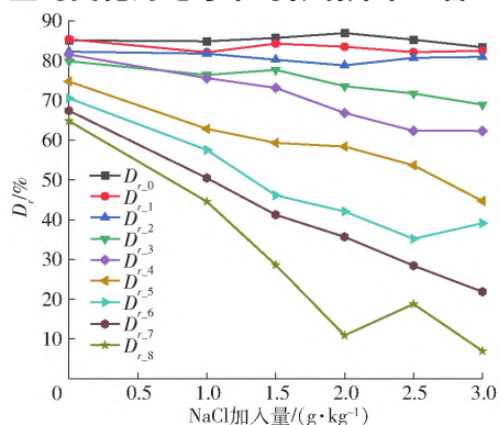
图 3 EC_0 与 EC_1 差值比 D_r 变化曲线
