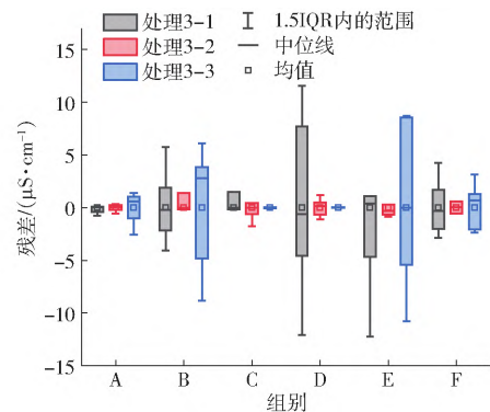
图6 处理3残差
