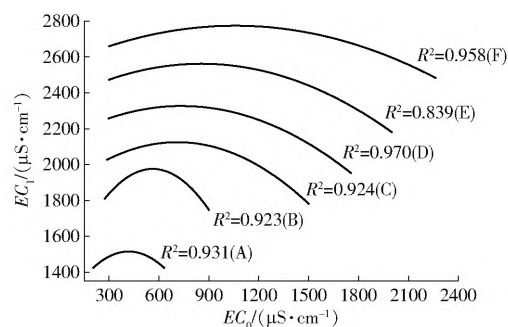
图 4 处理 1 的拟合结果
