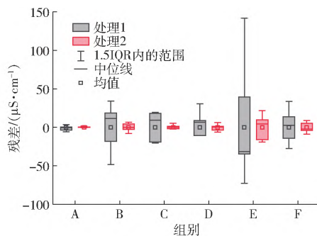
图5 处理1与处理2残差
