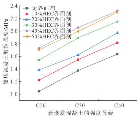
图 3 HEC 界面剂掺量及混凝土强度等级与混凝土劈拉强度关系图
