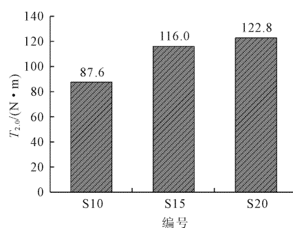
图10 钢纤维掺量对韧性的影响
