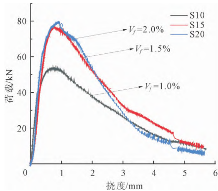
图7 不同钢纤维体积掺量 UHPC 荷载 - 挠度曲线
