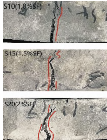
图6 不同纤维掺量的 UHPC 纯弯段裂缝形态
