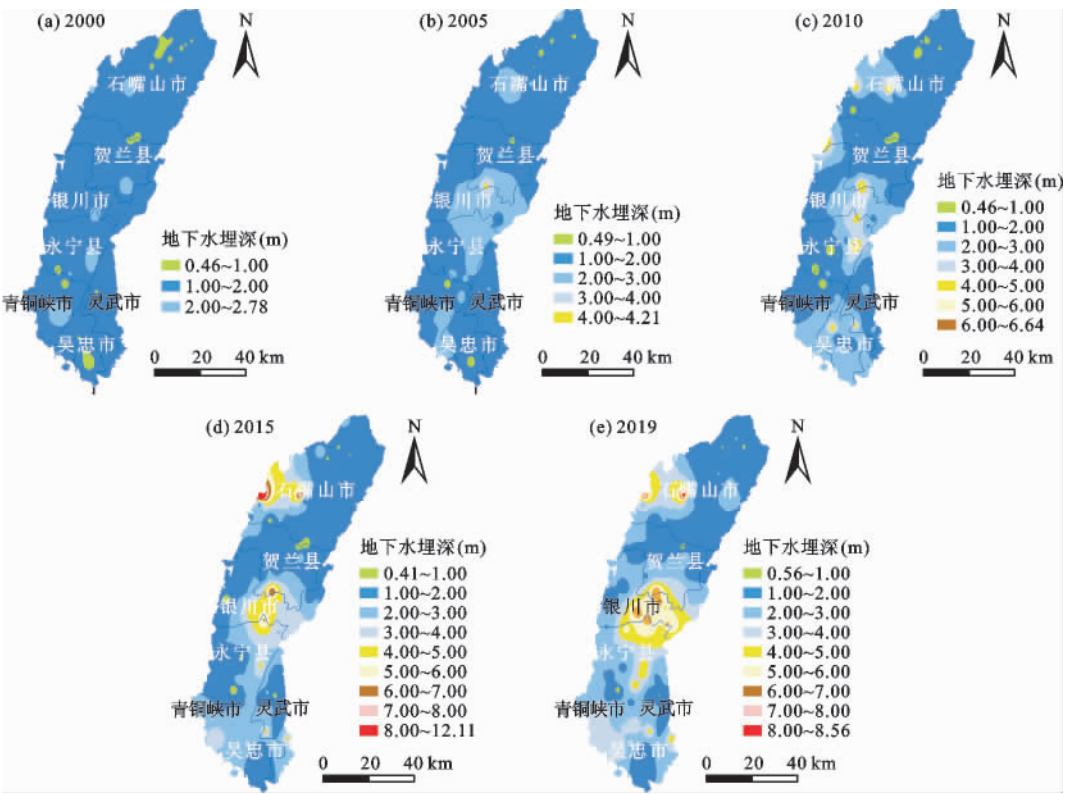
图 5 2000 – 2019 年银川平原地下水埋深时空动态
