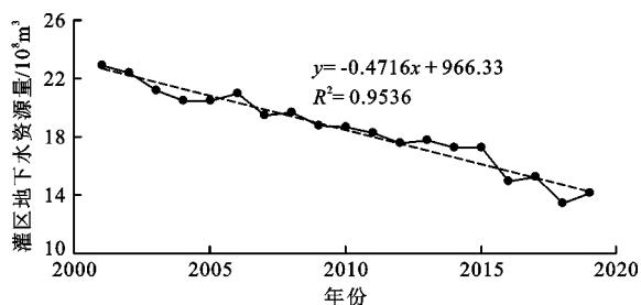
图 10 2001–2019 年宁夏引黄灌区地下水资源量变化
