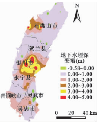
图 7 2000 – 2019 年银川平原地下水埋深不同变幅空间分布
